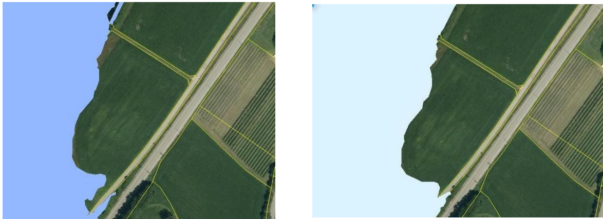
Überschwemmungsbereich eines 100 jährlichen Hochwasserereignisses in der Ilm, linkes Bild. Rechtes Bild, Überschwemmungsbereich der Ilm bei einem extremen Hochwasserereignis im Bereich der geplanten Photovoltaikanlage. Die baulichen Anlagen müssen außerhalb HQ100-Bereichs liegen. Daten: Bayerisches Landesamt für Umwelt, Bayerische Vermessungsverwaltung.
