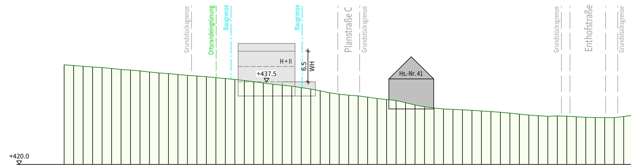
Geländeschnitt 4
